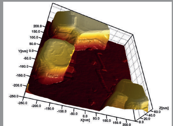
Imagine AFM în mod contact a filmului metalic cristalin cu structură insulară din imaginea alăturată (detaliu 200 nm x 200 nm)
