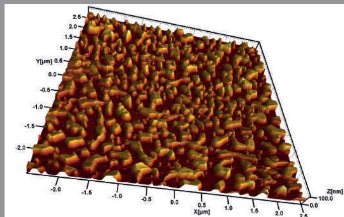
Imagine AFM în mod contact a unui film de Au cristalin cu structură insulară (2.5 μm x 2.5 μm)
