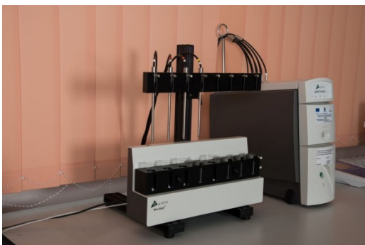
Sistem pentru monitorizarea in situ a vitezei de dizolvare μDISS Profiler
